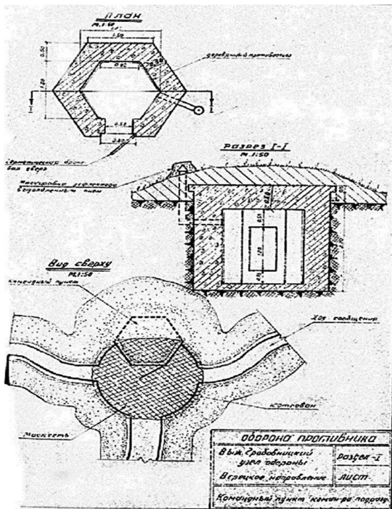
Рис. 3. Схема командного пункту командира підрозділу Верхньо-Гравіницького вузла оборони (Филоненко, 2017)
